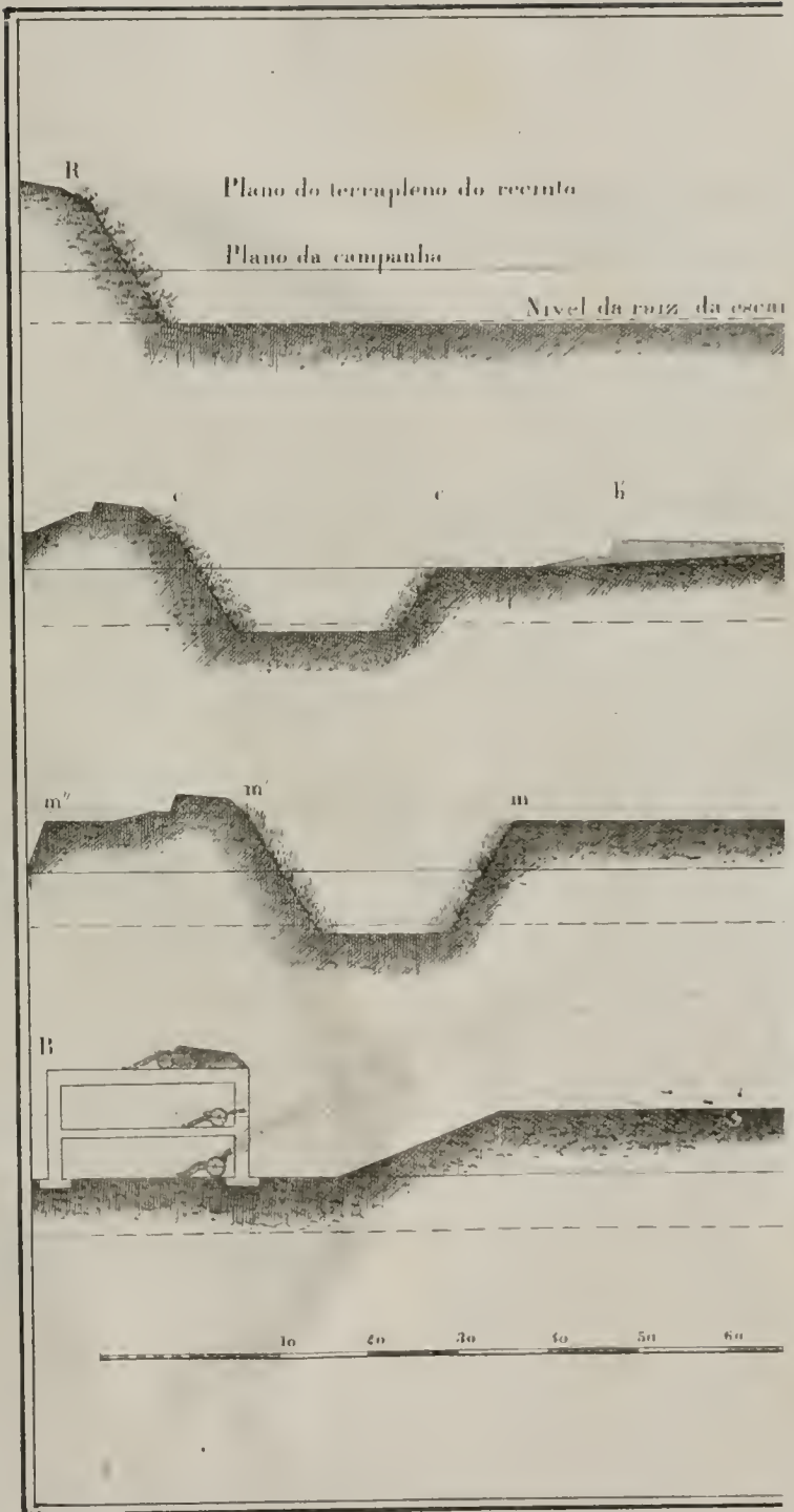
2º Systema portuguez 1855
